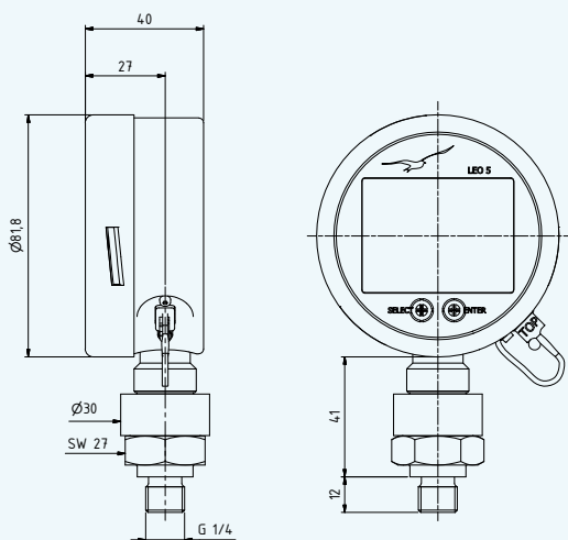
LEO5 manometer
